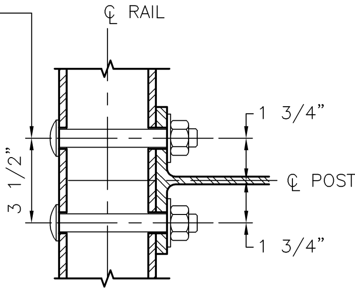
SECTION B-B SCALE: 3"=1'-0"
