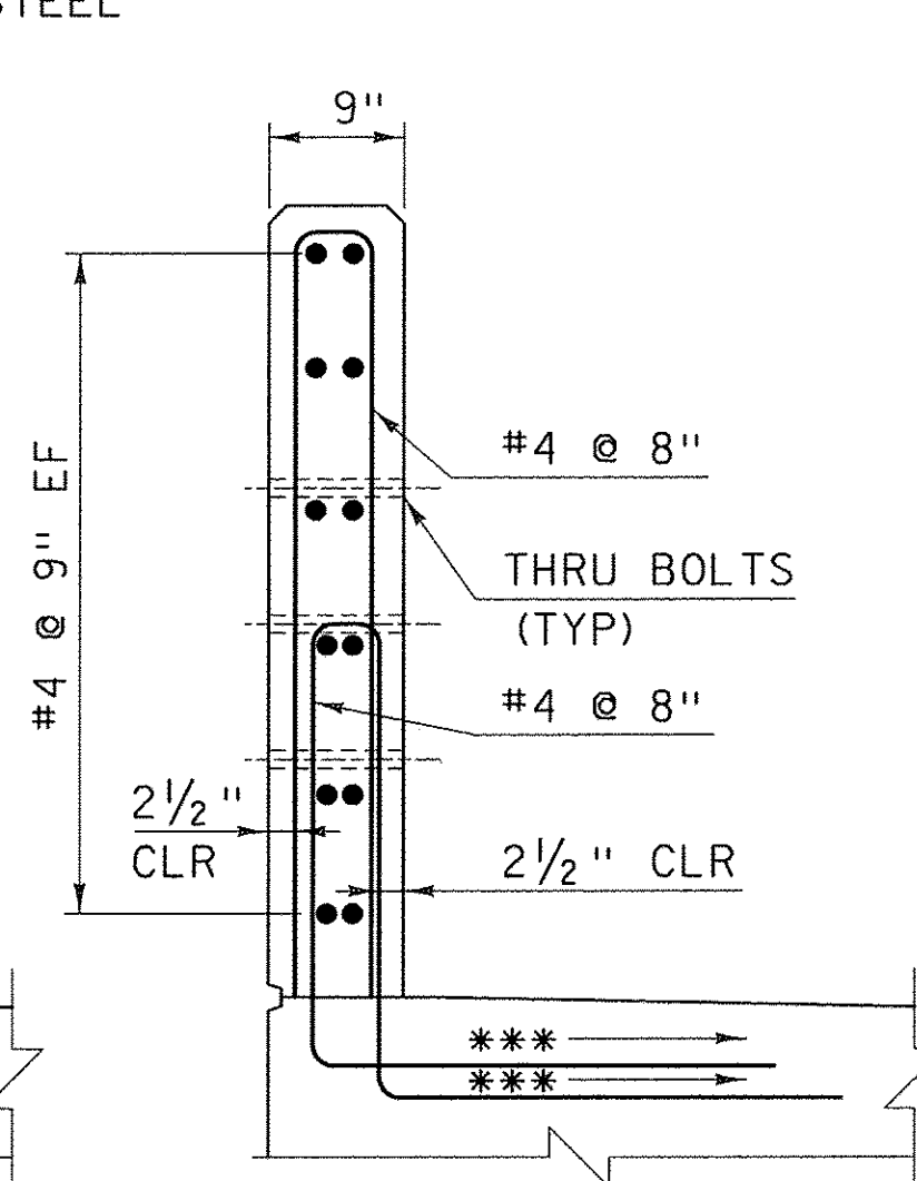
SECTION D-D
